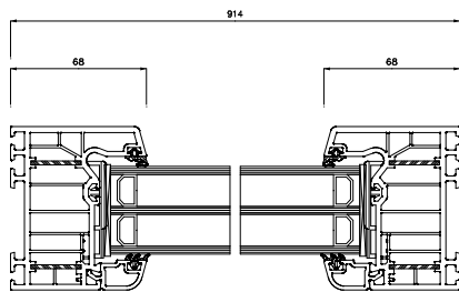
Schnitt S2(5:1)
