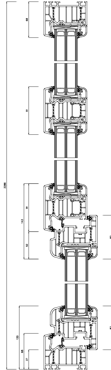
Schnitt S1(5:1)
