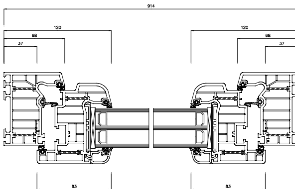
Schnitt S3(5:1)
