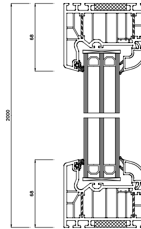
Schnitt S1(5:1)
