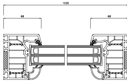
Schnitt S2(5:1)
