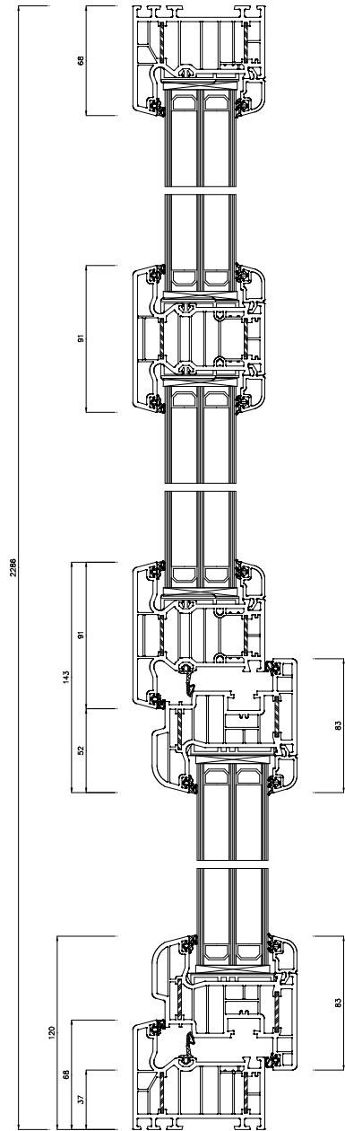
Schnitt S1(5:1)
