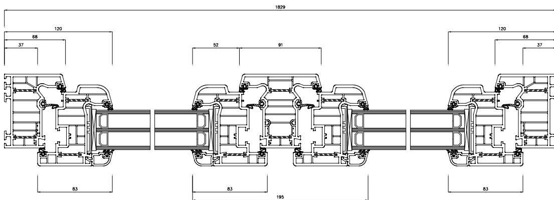
Schnitt S3(5:1)
