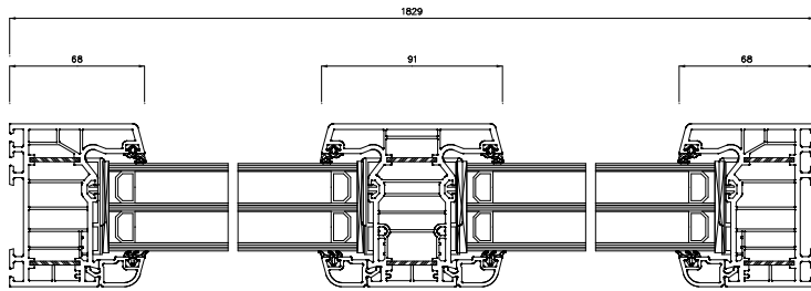
Schnitt S2(5:1)
