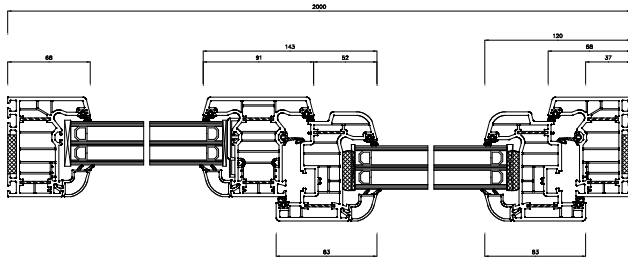
Schnitt S3(5:1)
