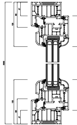
Schnitt S2(5:1)
