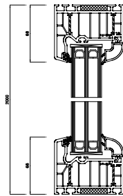
Schnitt S1(5:1)
