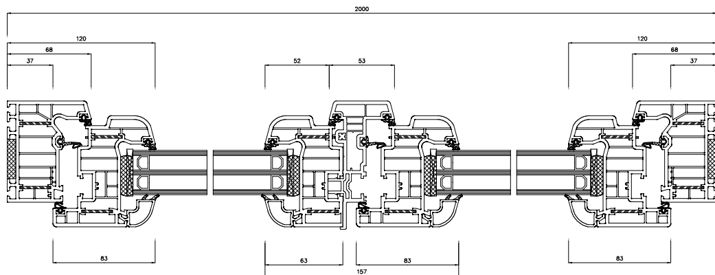
Schnitt S2(5:1)
