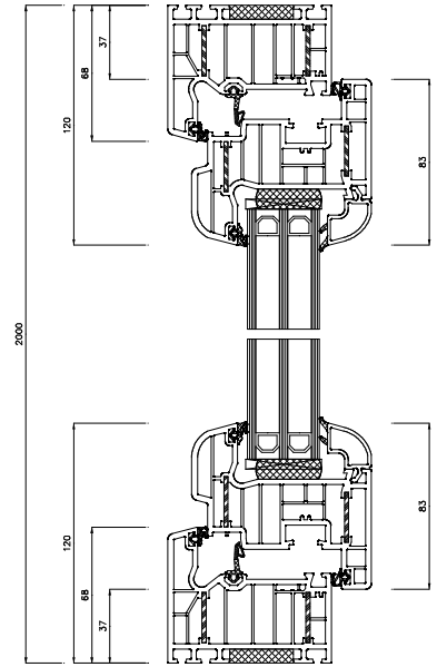
Schnitt S1(5:1)
