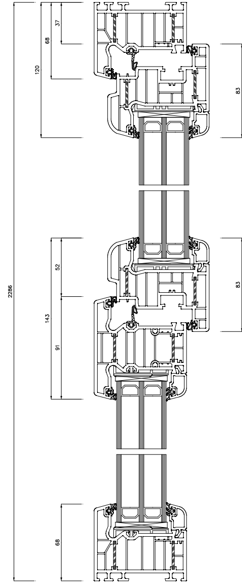
Schnitt S2(5:1)
