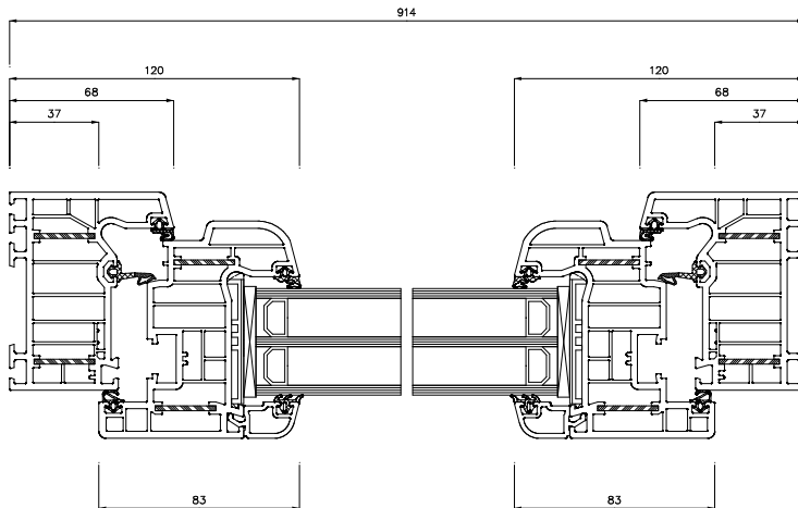
Schnitt S1(5:1)
