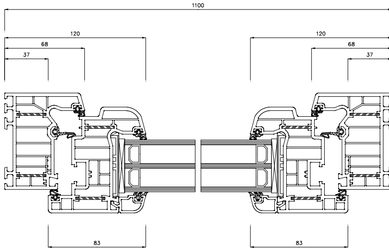
Schnitt S2(5:1)
