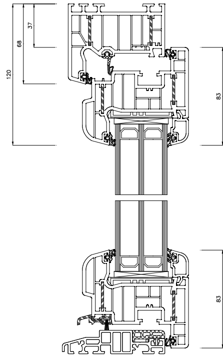
Schnitt S1(5:1)
