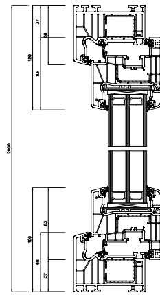
Schnitt S1(5:1)
