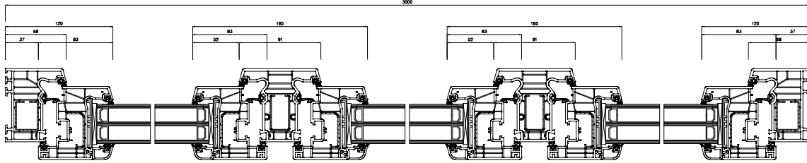
Schnitt S2(5:1)
