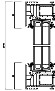
Schnitt S1(5:1)
