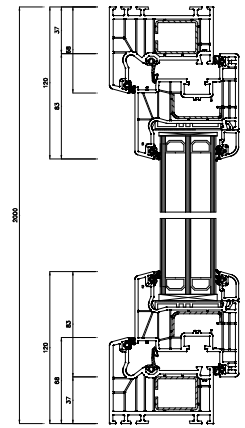
Schnitt S2(5:1)
