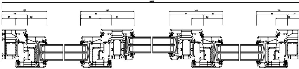
Schnitt S3(5:1)
