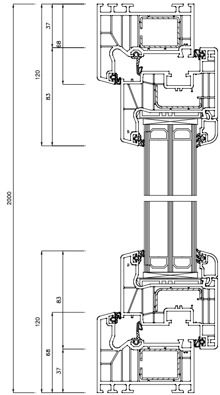
Schnitt S1(5:1)
