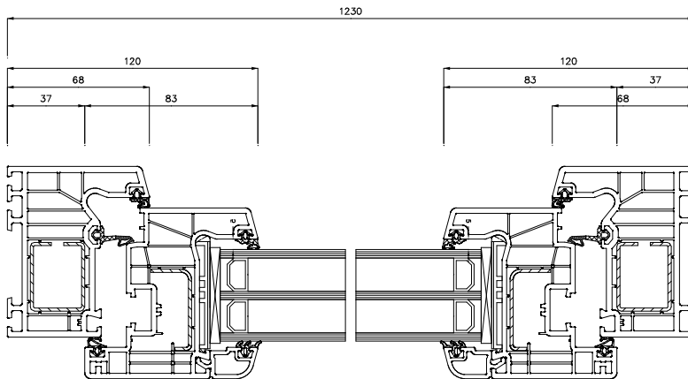
Schnitt S2(5:1)
