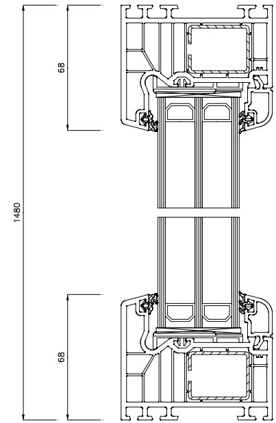
Schnitt S1(5:1)
