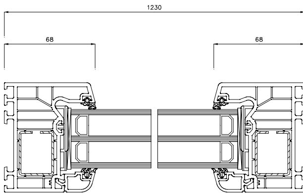
Schnitt S2(5:1)
