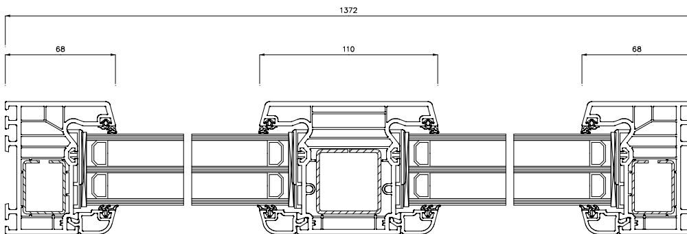
Schnitt S2(5:1)
