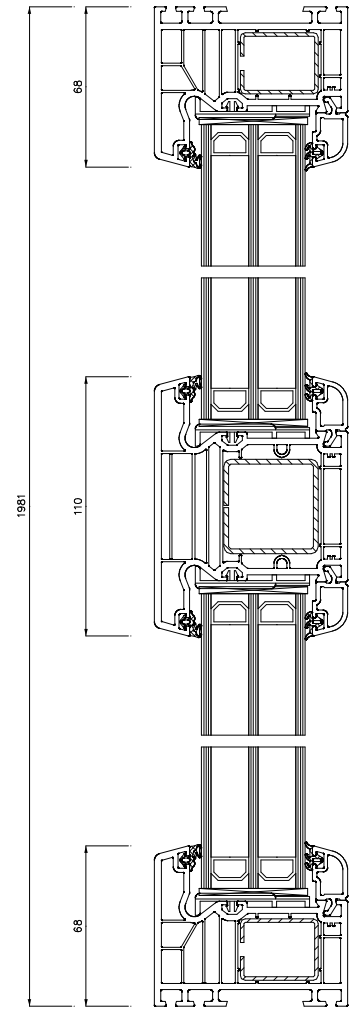
Schnitt S1(5:1)
