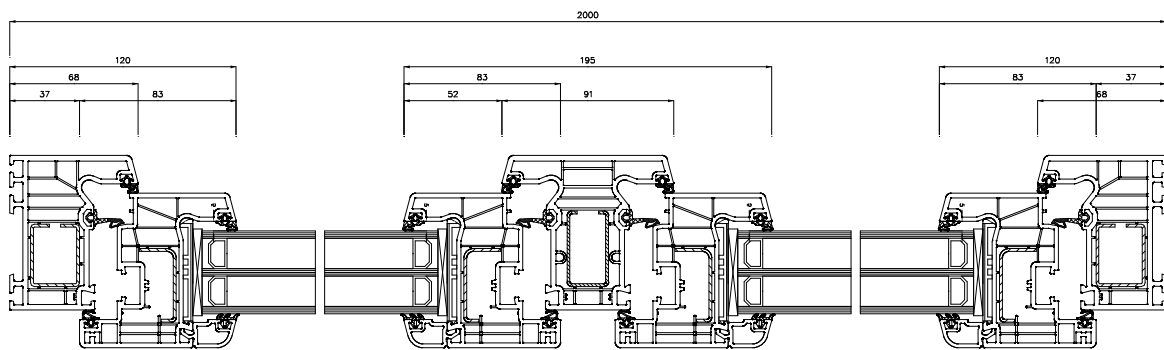
Schnitt S2(5:1)
