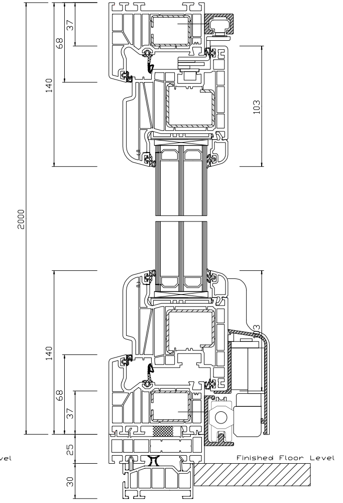
Schnitt S2(5:1)
