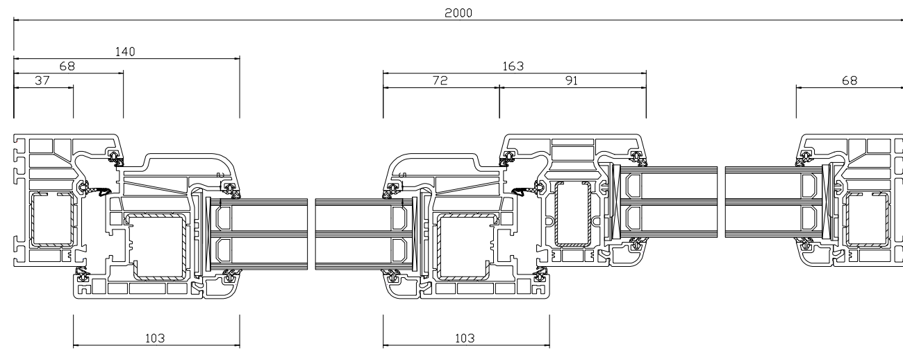
Schnitt S3(5:1)
