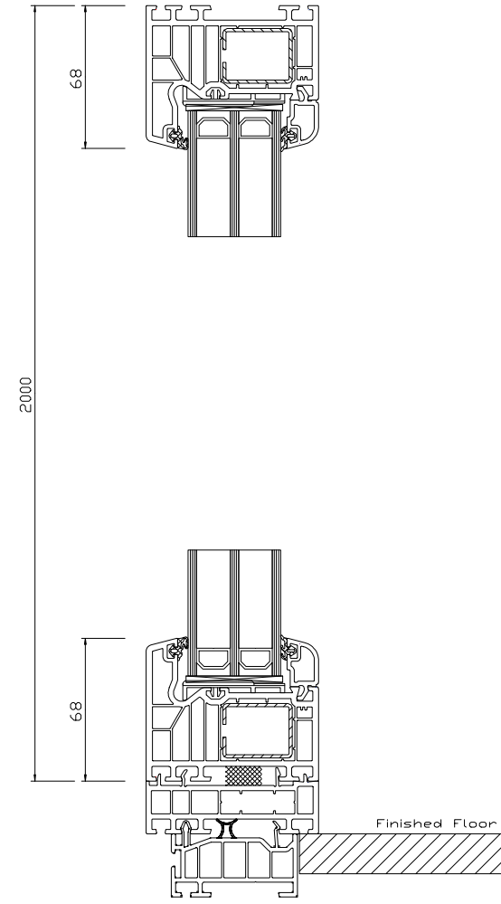
Schnitt S1(5:1)
