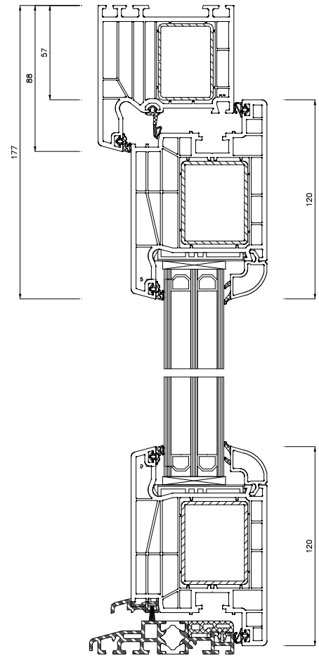
Schnitt S1(5:1)
