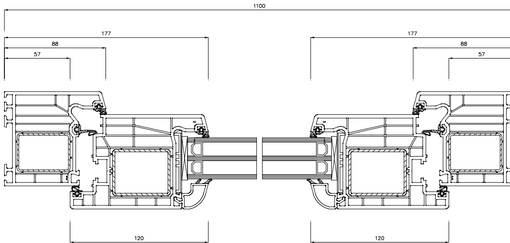
Schnitt S2(5:1)
