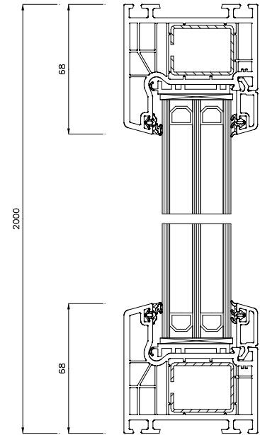
Schnitt S1(5:1)
