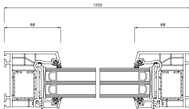
Schnitt S2(5:1)
