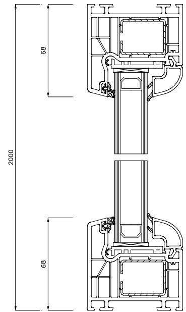
Schnitt S1(5:1)
