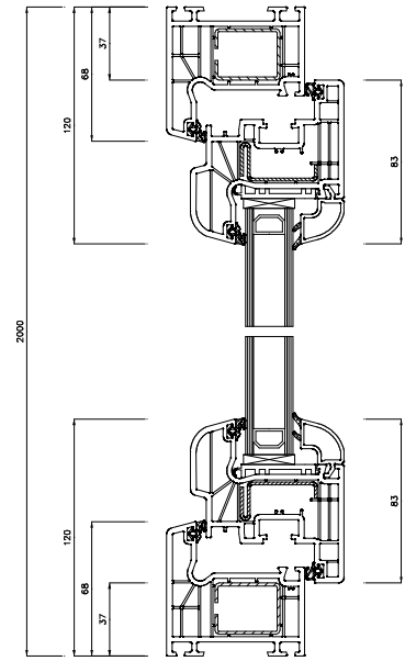
Schnitt S1(5:1)
