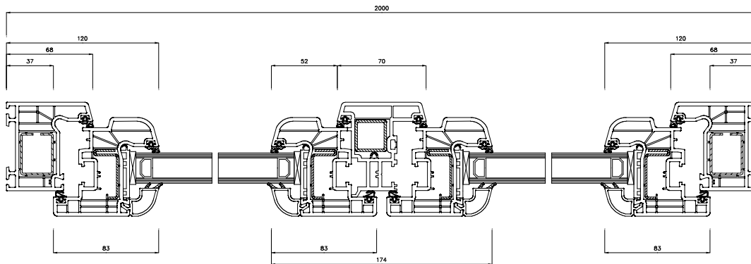
Schnitt S2(5:1)
