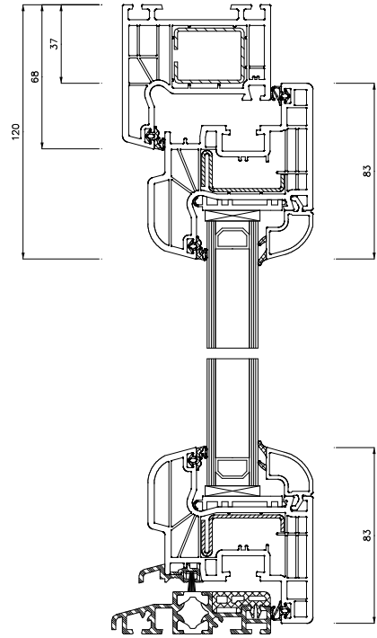
Schnitt S1(5:1)
