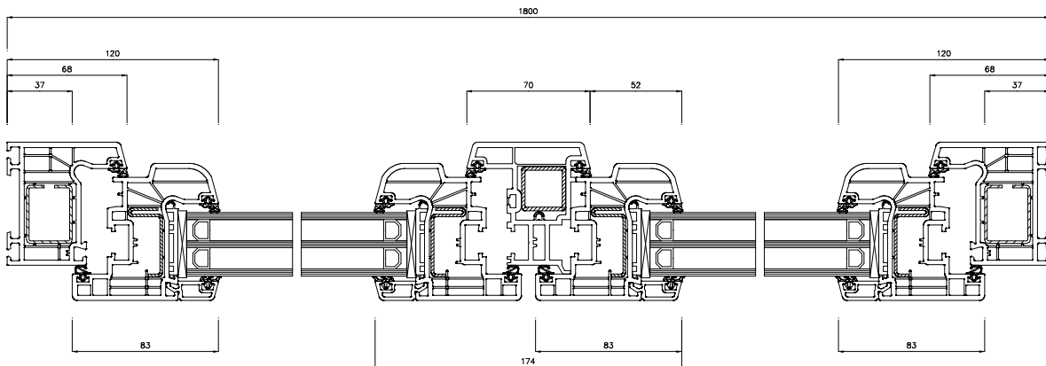
Schnitt S2(5:1)
