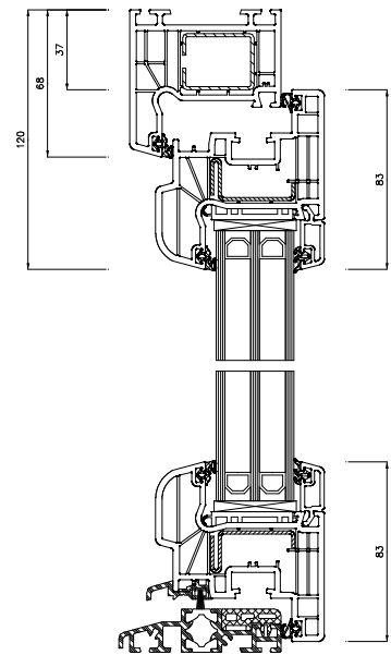
Schnitt S1(5:1)
