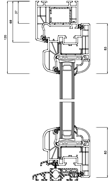
Schnitt S1(5:1)
