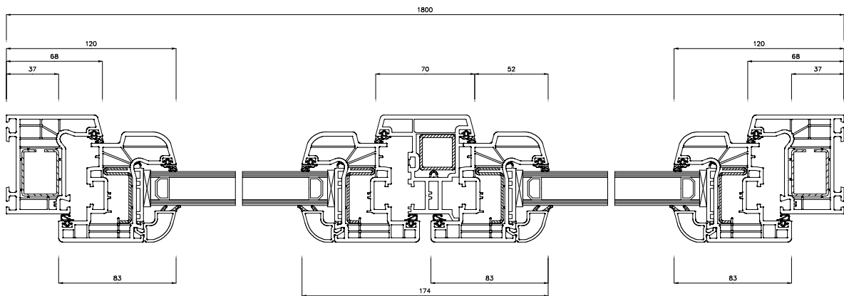
Schnitt S2(5:1)
